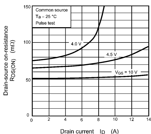
Fig. 8.4 RDS(ON) - ID
