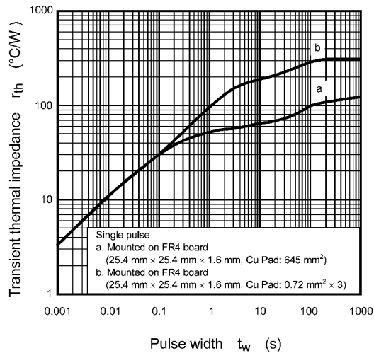
Fig. 7.13 r_{th} - t_w
