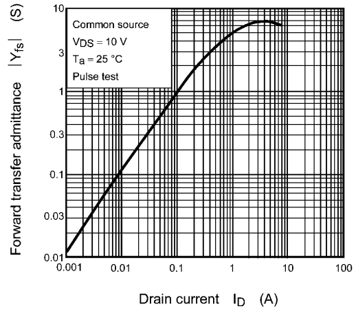
Fig. 7.8 |Y_{fs}| - I_D
