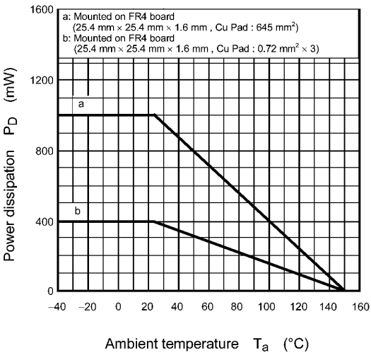
Fig. 7.14 P_D - T_a
