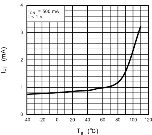
Fig. 14.1.6 I_{FT} - T_a
