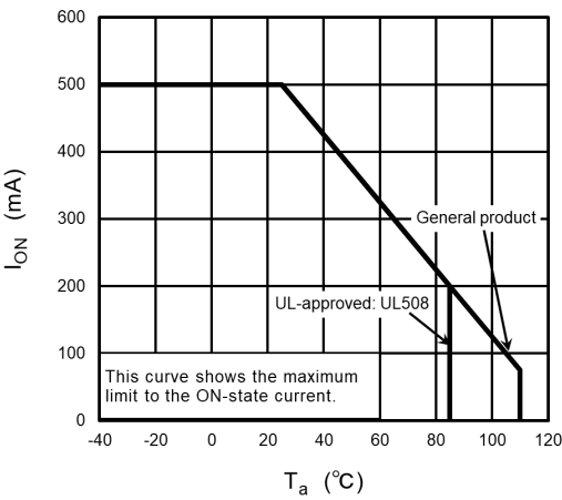
Fig. 14.1.2 I_{ON} - T_a
