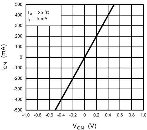
Fig. 14.1.4 I_{ON} - V_{ON}
