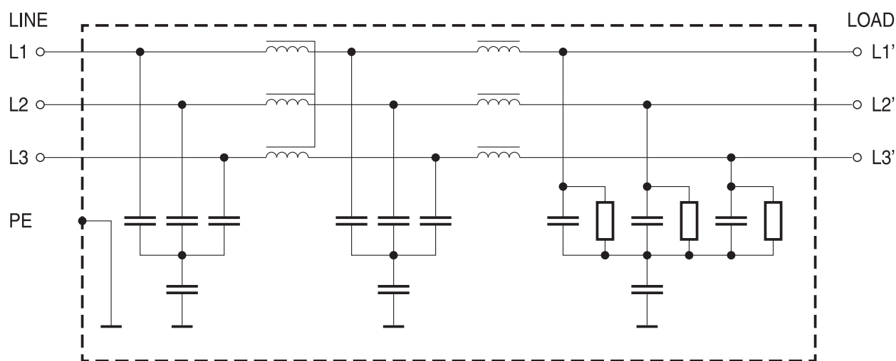
B84143B*S08*
