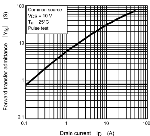
Fig. 8.5 |Y_{fs}| - I_D
