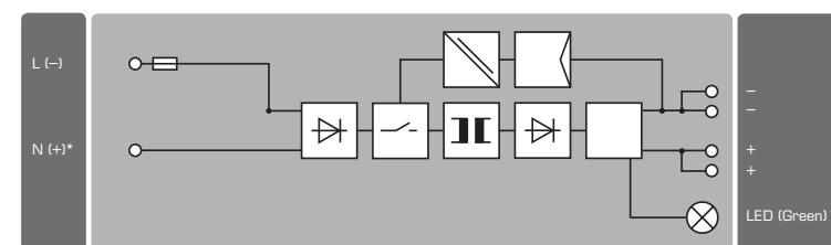
Funktionsschaltbild für PEL 230 Functional diagram for PEL 230
