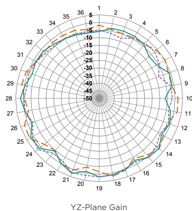
YZ-Plane Gain
