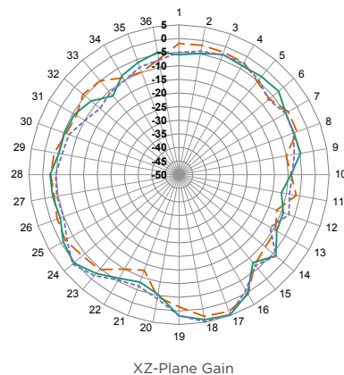
XZ-Plane Gain
