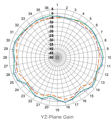
YZ-Plane Gain
