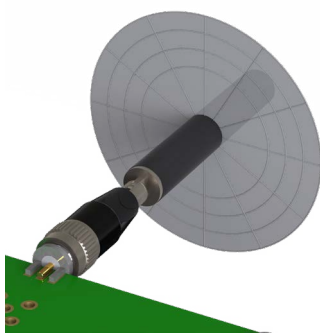
XZ-Plane Gain
