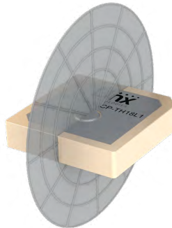
YZ-Plane Gain
