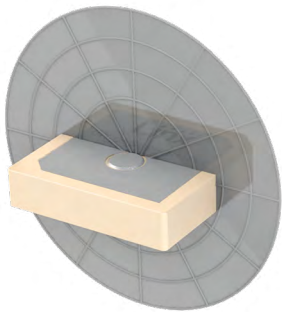
XZ-Plane Gain
