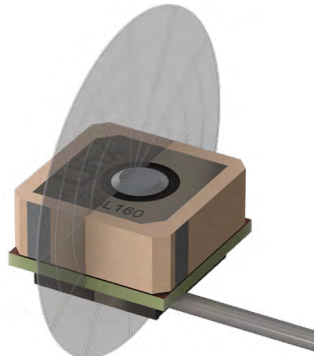
YZ-Plane Gain
