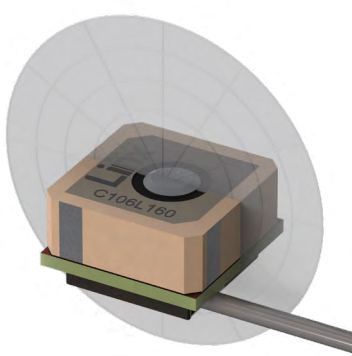
XZ-Plane Gain
