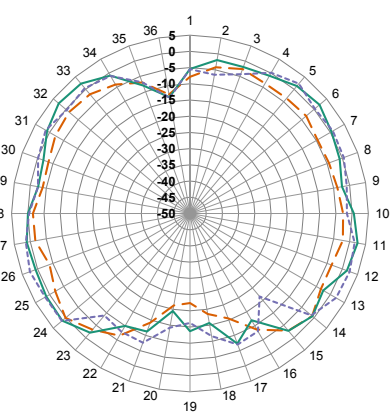
YZ-Plane Gain
