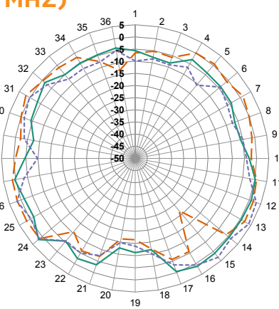
YZ-Plane Gain
