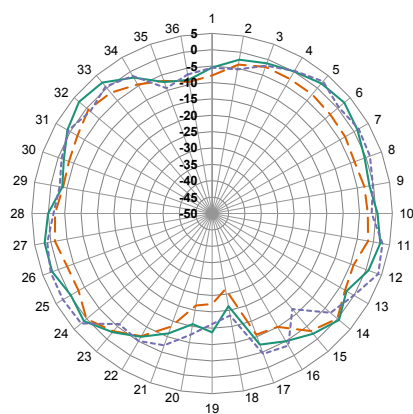
XZ-Plane Gain
