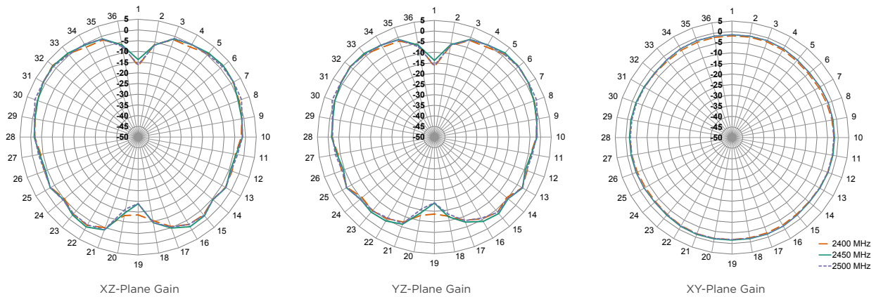
XZ-Plane Gain
