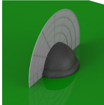
YZ-Plane Gain
