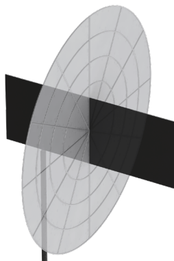
YZ-Plane Gain
