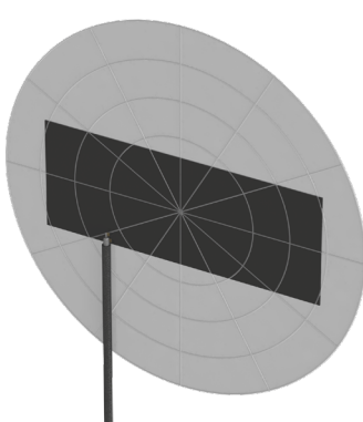
XZ-Plane Gain
