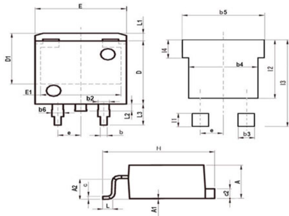
TO-263S, (TO-263S)
