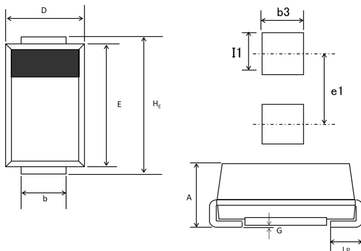
DO-214AC(SMA)
