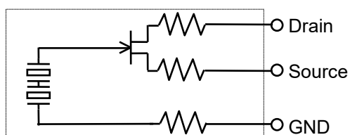
図3. 内部回路構成
