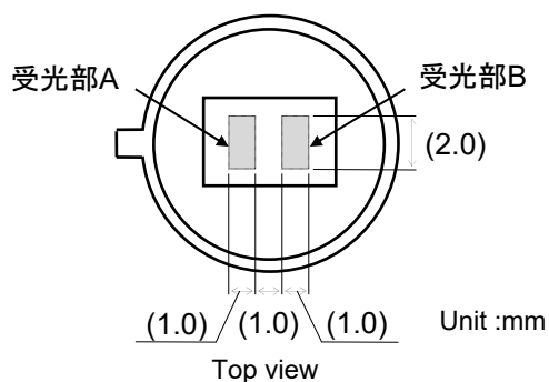
図 2. 受光部寸法
