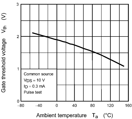
Fig. 8.9 V_{th} - T_a
