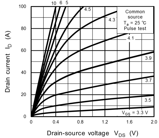
Fig. 8.2 I_D - V_{DS}
