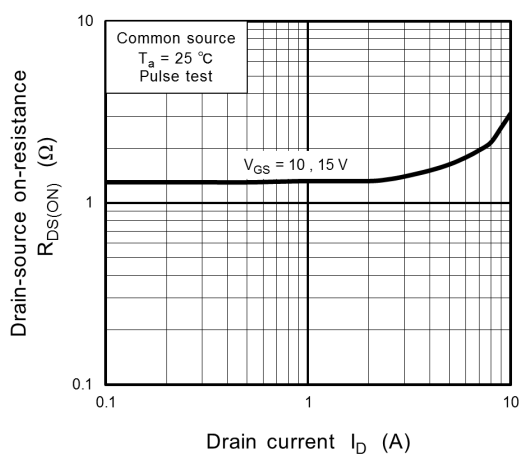
Fig. 8.6 R_{DS(ON)} - I_D
