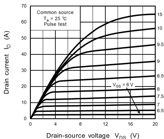
Fig. 8.2 I_D - V_{DS}
