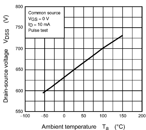
Fig. 8.5 V_{DS} - T_a
