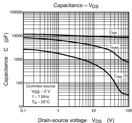
Fig. 8.8 Capacitance - V_{DS}
