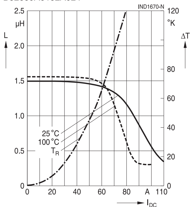
B82559A3152A024
