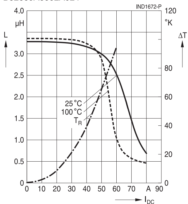
B82559A5332A024
