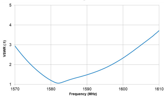
VSWR
