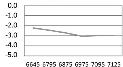
6645MHz~7125MHz
