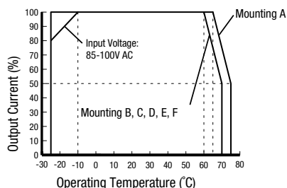
PS5R-VB05, -VB12, -VB24
