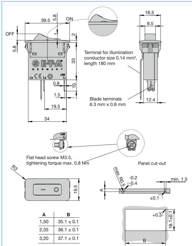
Dimensions 3130-F120-...
