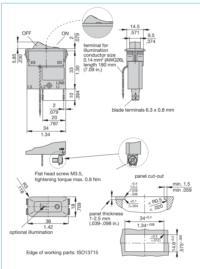
Dimensions 3130-F110-...
