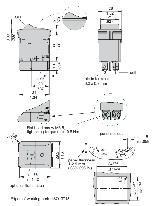
Dimensions 3130-F120-...
