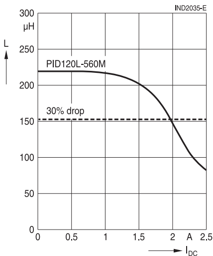
PID120L-560M
