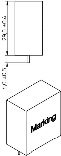
Scale - 1:1
