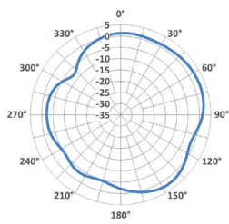
Horizontal - 3500 MHz
