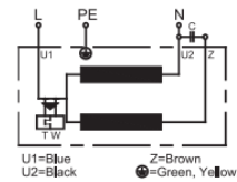
MOTOR WIRING DIAGRAMS
