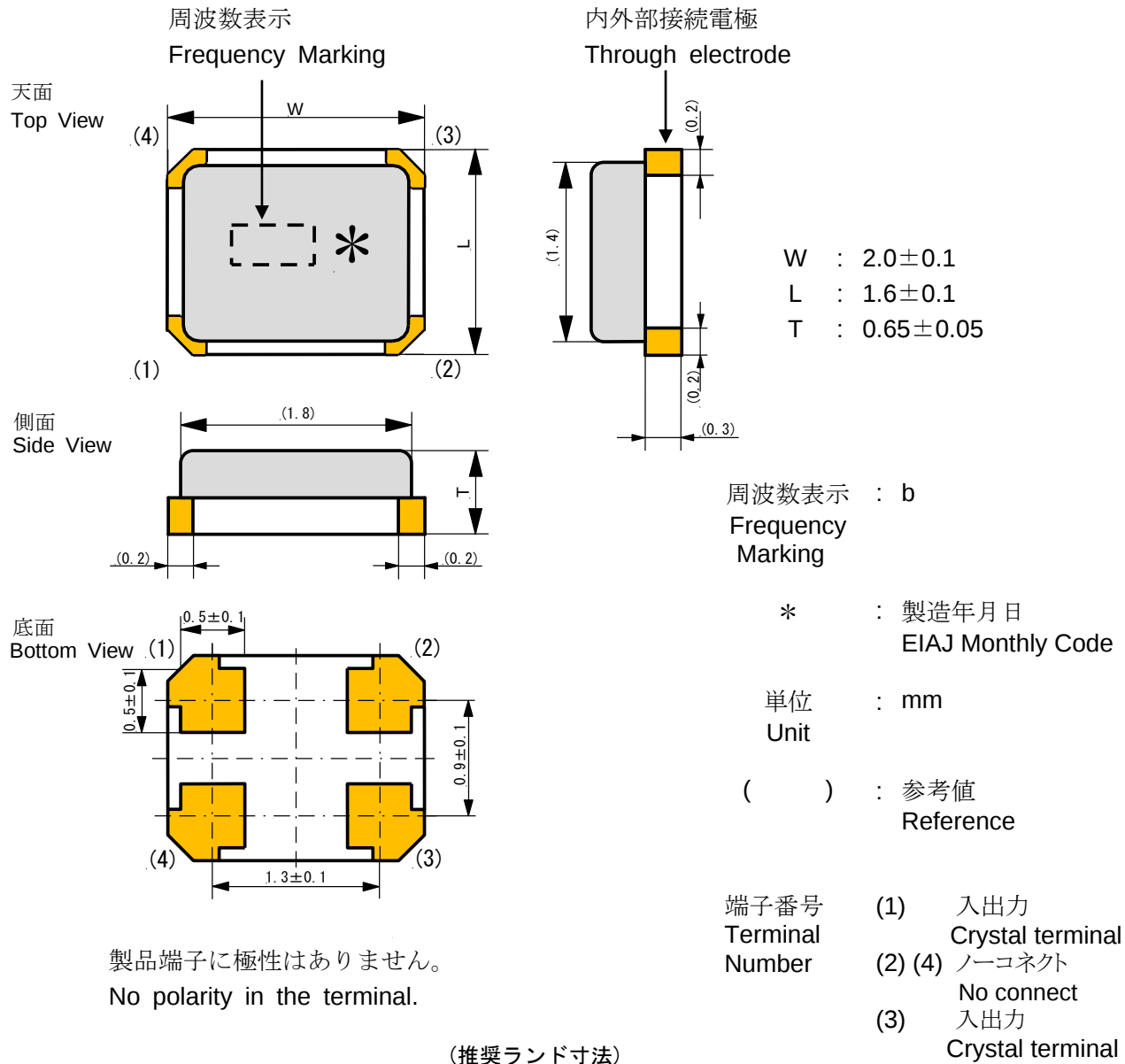
(推奨ランド寸法) (Recommendable Land Pattern)
