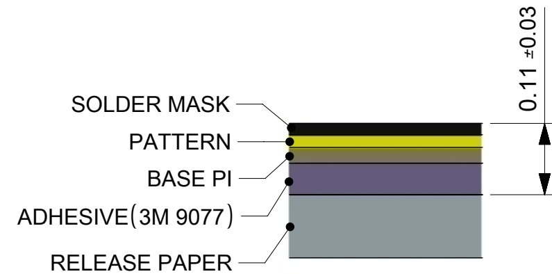
DETAIL B SCALE 120:1 FLEX LAYER
