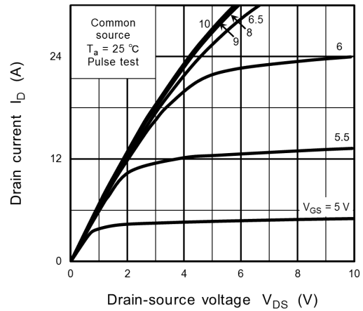
Fig. 8.2 I_D - V_{DS}
