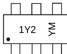
SOT363
