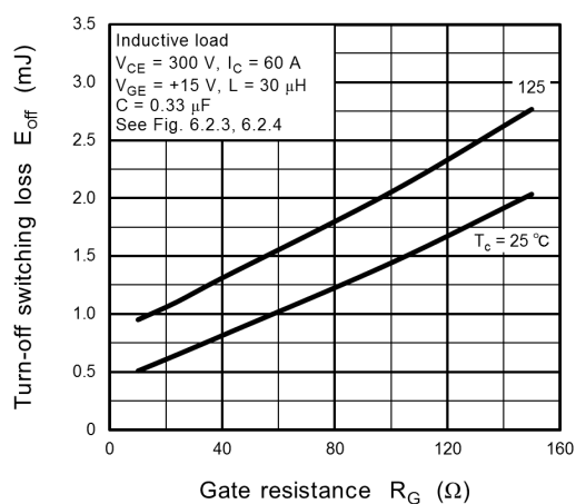
Fig. 8.16 E_{off} - R_G
