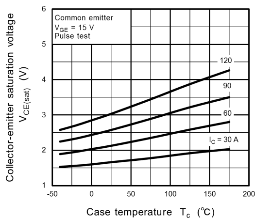
Fig. 8.5 V_{CE(sat)} - T_c
