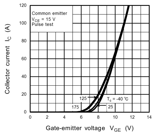
Fig. 8.6 I_C - V_{GE}
