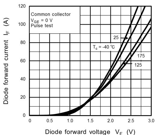
Fig. 8.11 I_F - V_F
