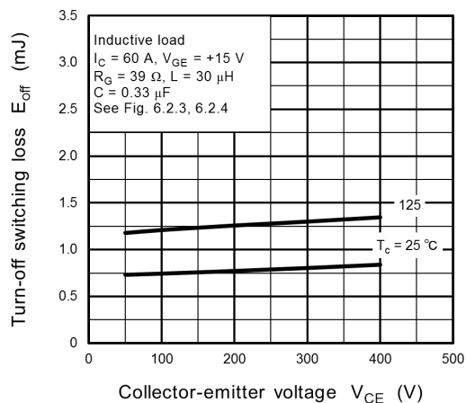
Fig. 8.14 E_{off} - V_{CE}
