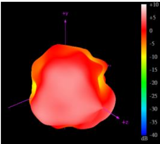
5150MHz
