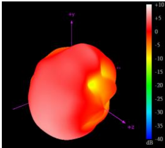
2400MHz
