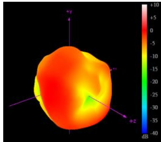
2690MHz
