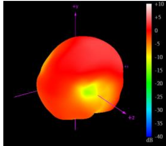
2170MHz
