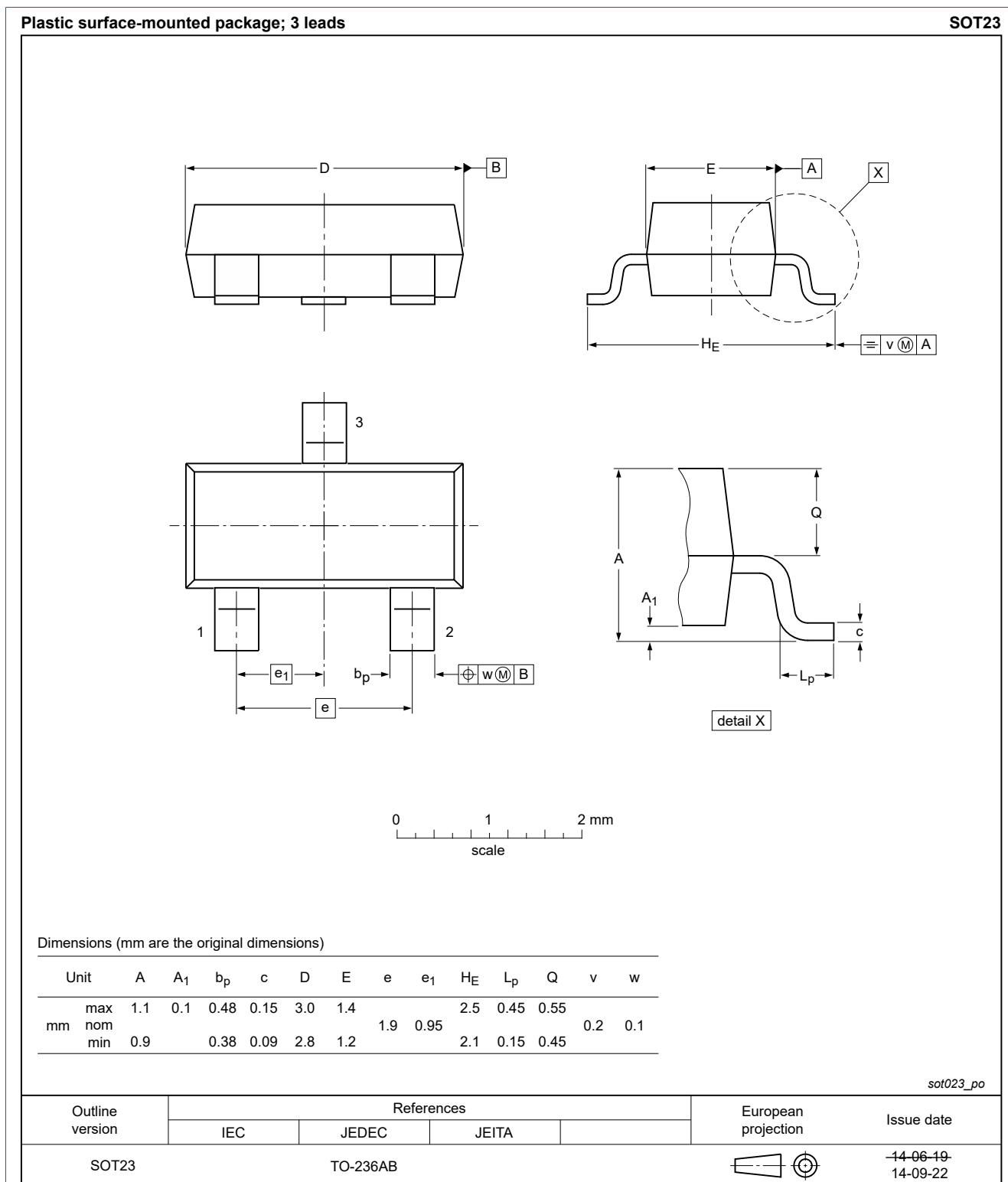
Fig. 18. Package outline SOT23
