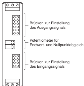
Abbildung 3 Frontansicht mit geöffneter Abdeckung
