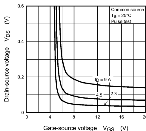
Fig. 8.4 V_{DS} - V_{GS}
