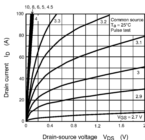
Fig. 8.2 I_D - V_{DS}
