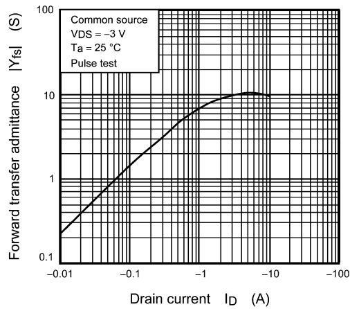
Fig. 8.7 |Y_{fs}| - I_D
