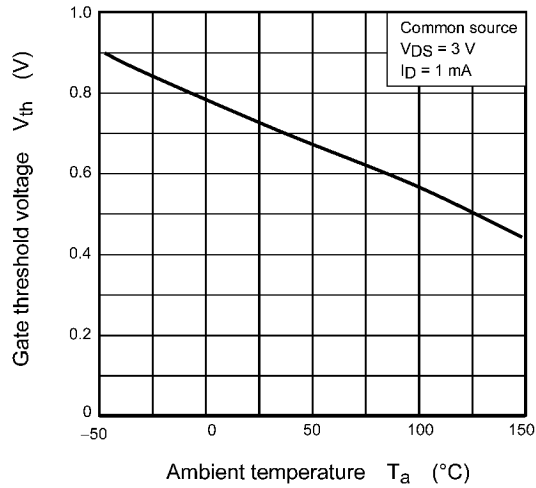
Fig. 7.7 V_{th} - T_a
