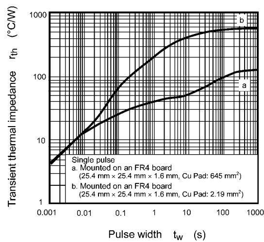
Fig. 7.13 r_{th} - t_w
