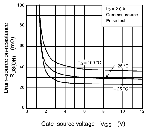
Fig. 7.4 R_{DS(ON)} - V_{GS}
