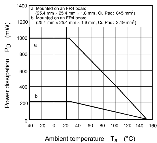
Fig. 7.14 P_D - T_a
