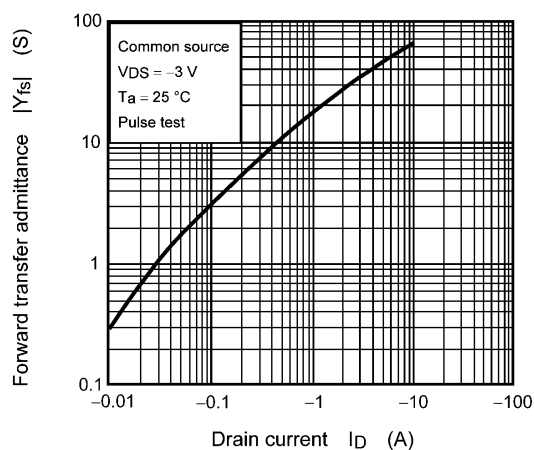
Fig. 8.8 |Y_{fs}| - I_D
