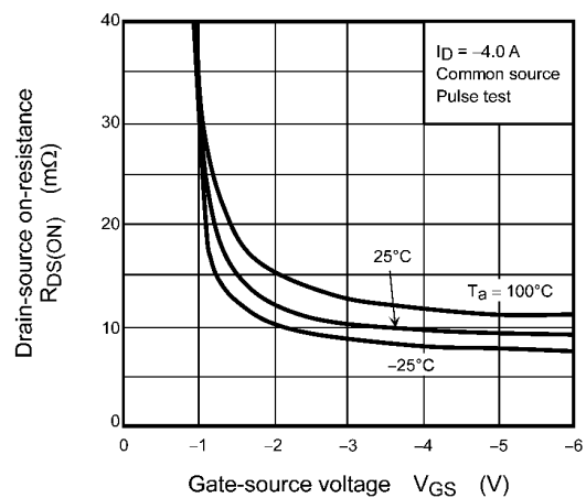
Fig. 8.4 R_{DS(ON)} - V_{GS}
