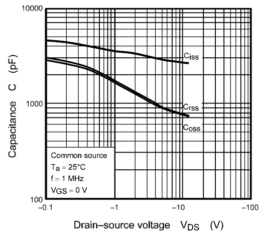
Fig. 8.10 C - V_{DS}
