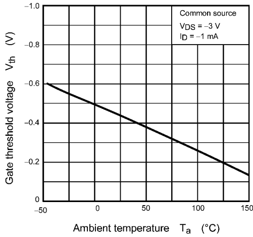
Fig. 8.7 V_{th} - T_a
