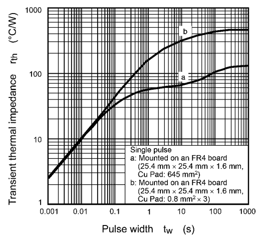
Fig. 8.12 r_{th} - t_w
