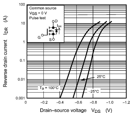
Fig. 8.9 I_{DR} - V_{DS}
