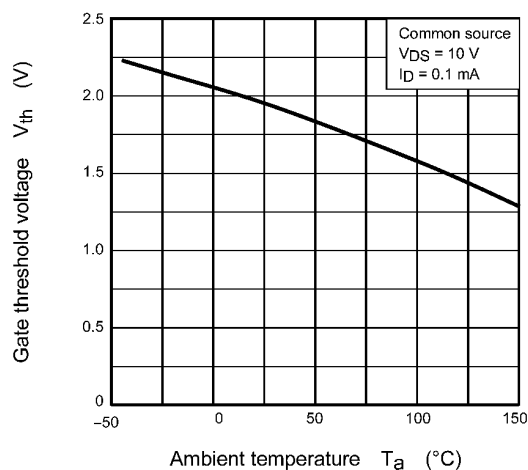
Fig. 8.7 V_{th} - T_a
