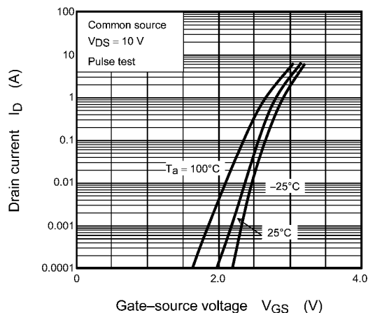
Fig. 8.2 I_D - V_{GS}
