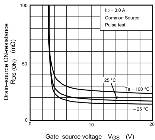
Fig. 7.3 R_{DS(ON)} - V_{GS}
