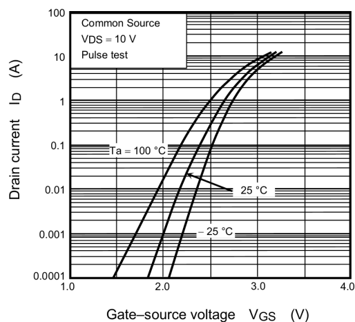
Fig. 7.2 I_D - V_{GS}
