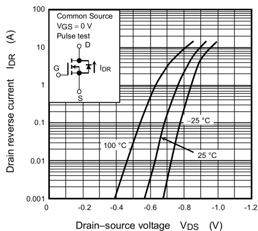
Fig. 7.7 I_{DR} - V_{DS}
