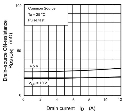
Fig. 7.4 R_{DS(ON)} - I_D
