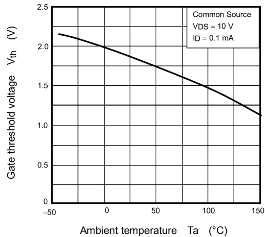
Fig. 7.6 V_{th} - T_a
