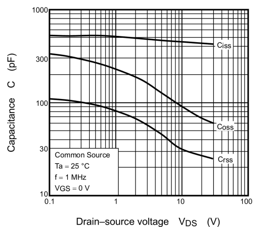
Fig. 7.8 C - V_{DS}
