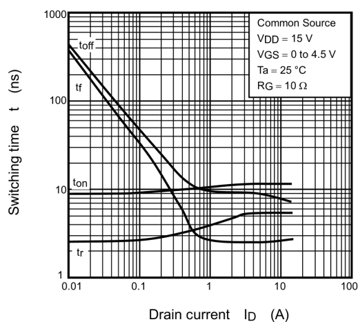
Fig. 7.9 t - I_D
